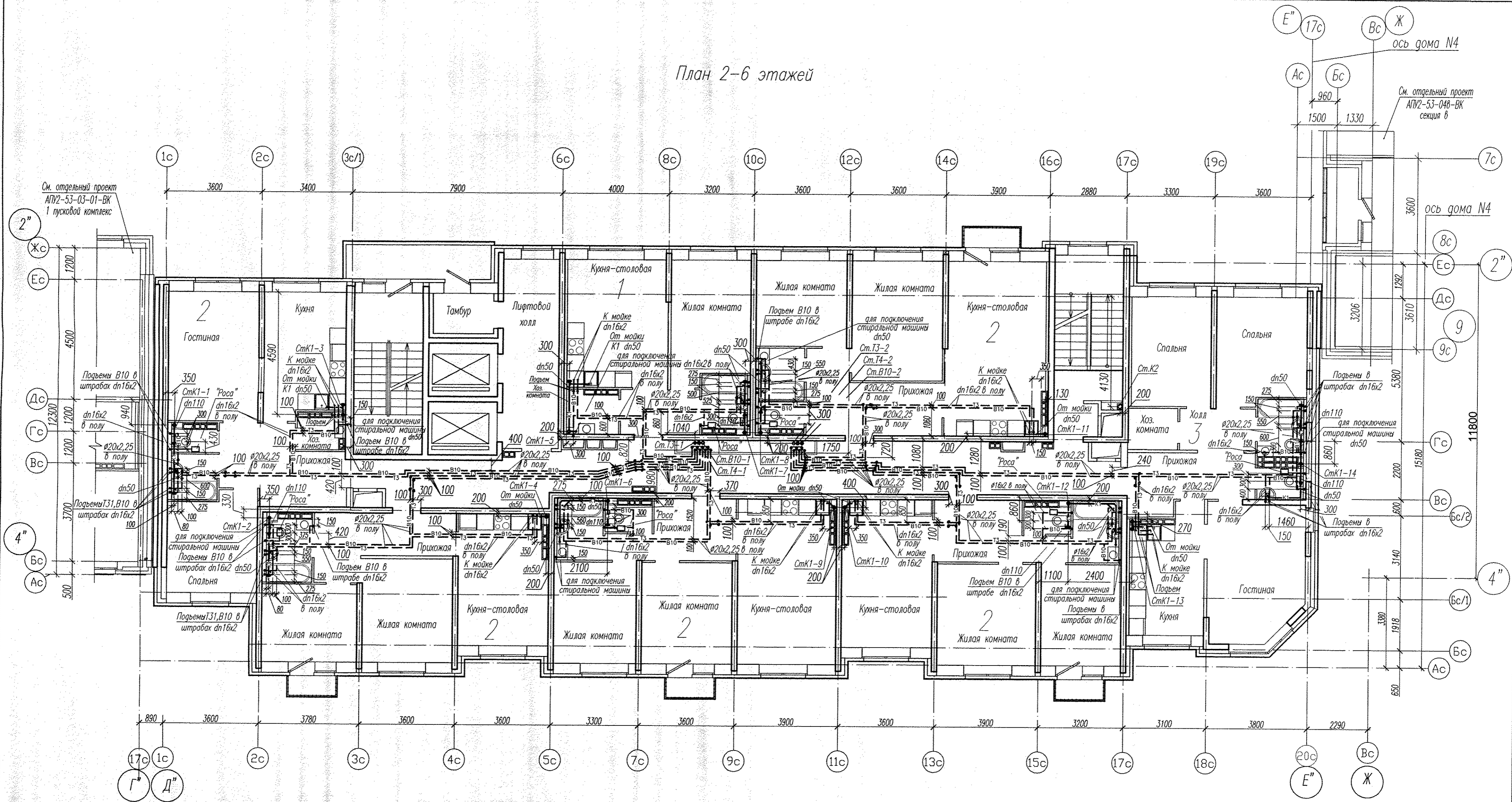
Компоновочная схема
